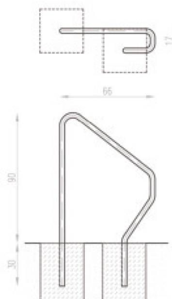
Versie met verlengde buis voor instorten met beton
