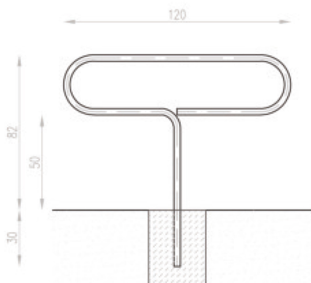
Versie met verlengde buis voor instorten met beton
