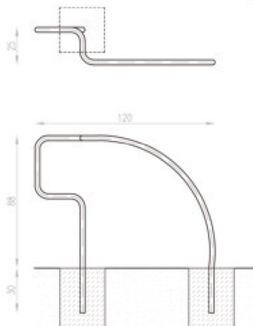
Versie met verlengde buis voor instorten met beton
